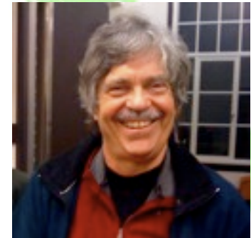
Alan Kay
